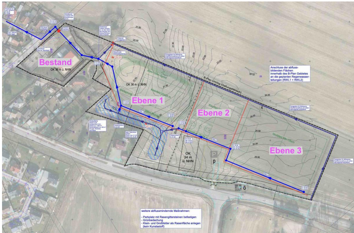
Abbildung 4: Auszug aus dem Entwässerungskonzept (Ingenieurbüro Voss & Muderack)
